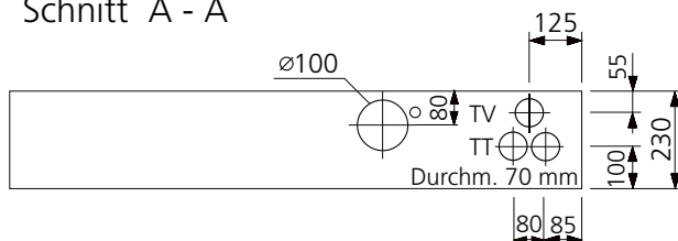
Schnitt A - A
